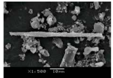
Stark geschädigte Fasern aus realem Brandfall
